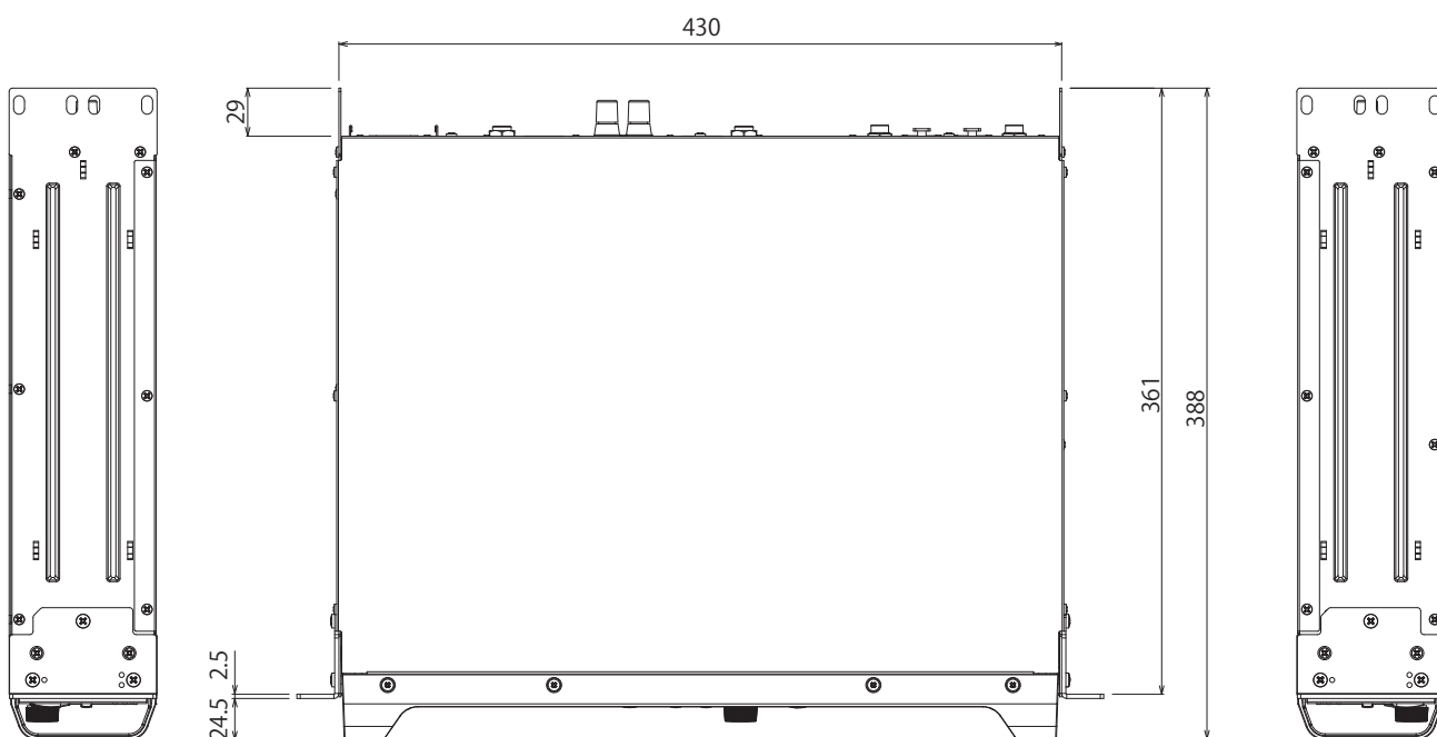
左側面図
